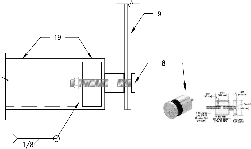
D STANDOFF STEEL CONN. DETAIL SD3.3 SCALE: 3"=1'-0"
