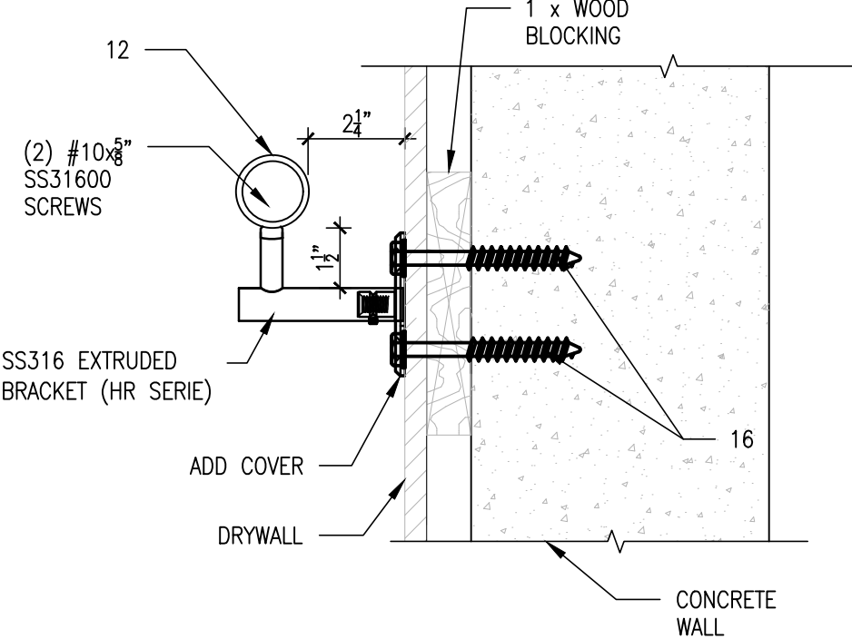
C CONN DETAIL SD3.3 SCALE: 3"=1'-0"
