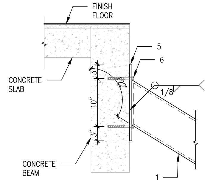
D TOP CONN. DETAIL SD3.0 SCALE: 1"=1'-0"
