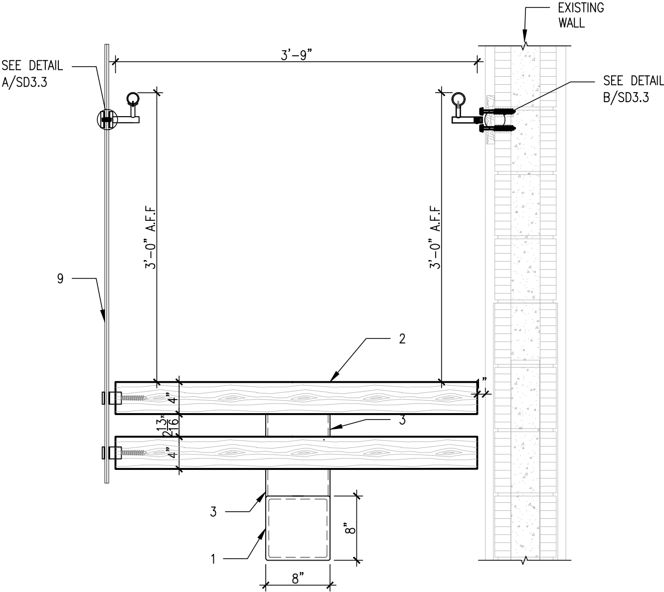
3 STAIR SECTION SD3.2 SCALE: 1"=1'-0"
