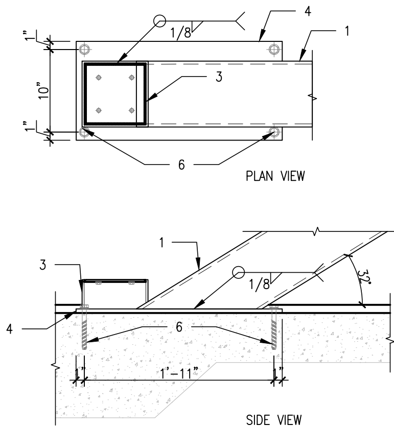
A BOTTOM. CONN. DETAIL SD3.0 SCALE: 1"=1'-0"
