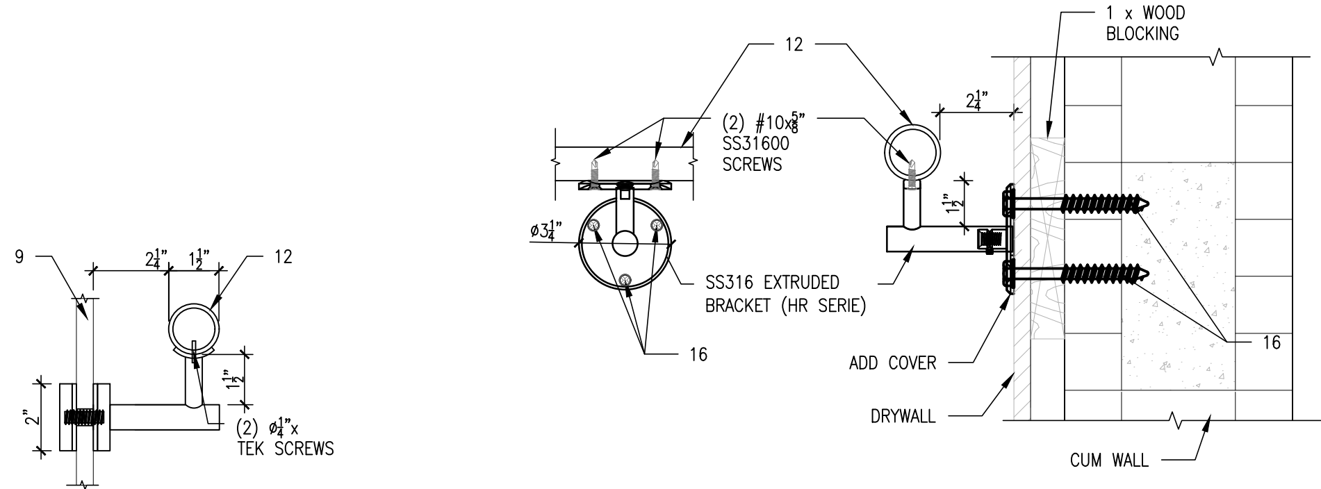
A BRACKET DETAIL SD3.3 SCALE: 3"=1'-0"
